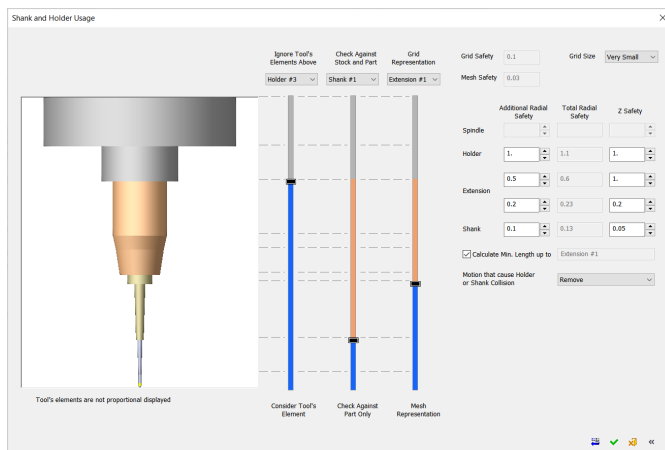
Un nuevo diálogo para el mango y portaherramientas permite un mayor control al usuario e información completamente transparente sobre los distintos componentes del montaje de una herramienta, considerándolos o ignorándolos, para una mayor seguridad con un feedback interactivo completo.
