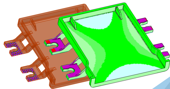
Desviación entre la pieza moldeada y la pieza modelada reconocida y compensada.
