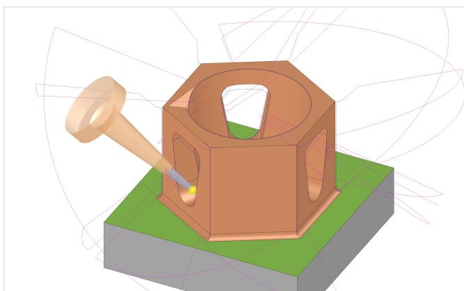
Imagen de un desbarbado en 5X, calculado automáticamente sobre las aristas vivas de pieza.
