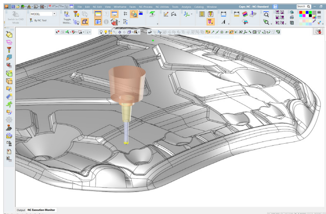
Imagen de acabado de utillaje usando una herramienta de sección circular de diámetro 20mm, el tiempo de mecanizado se vió reducido un 10%, de 132 horas a 119 comparándolo con una herramienta esférica convencional.
