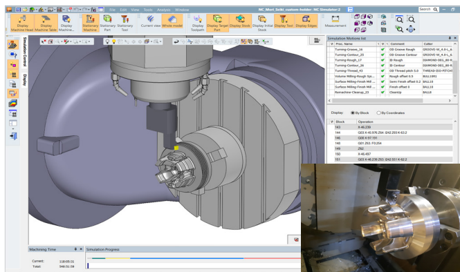
Nueva aplicación de Mill/Turn integrada completamente en el entorno CAM de Cimatron
