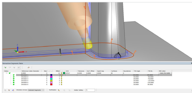
Imagen de un remecanizado de una esquina, mecanizada en una orientación inclinada en 3x+2x . La orientación ha sido calculada automáticamente por el sistema, como parte de la función de autoinclinación dentro del remecanizado guiado.
