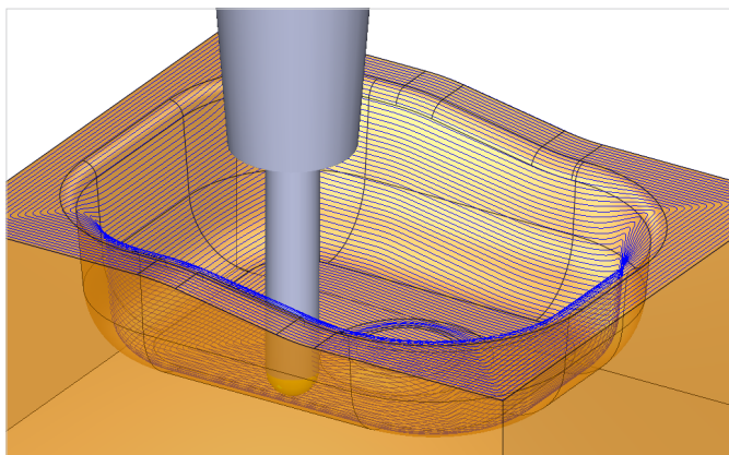
Trayectoria en paso 3D Geodésico en 3 ejes sobre una cavidad de un molde, sin reentradas, para conseguir la mayor calidad superficial posible sin marcas de entradas y salidas.
